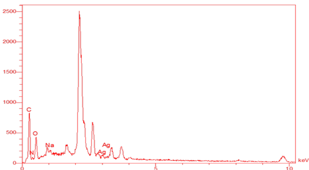
Fig. 11. EDS spectrum.
